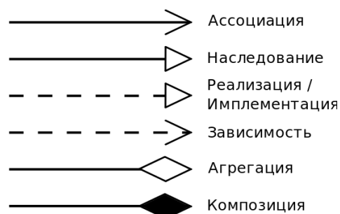
Рис. 6.2. Виды отношений между классами
