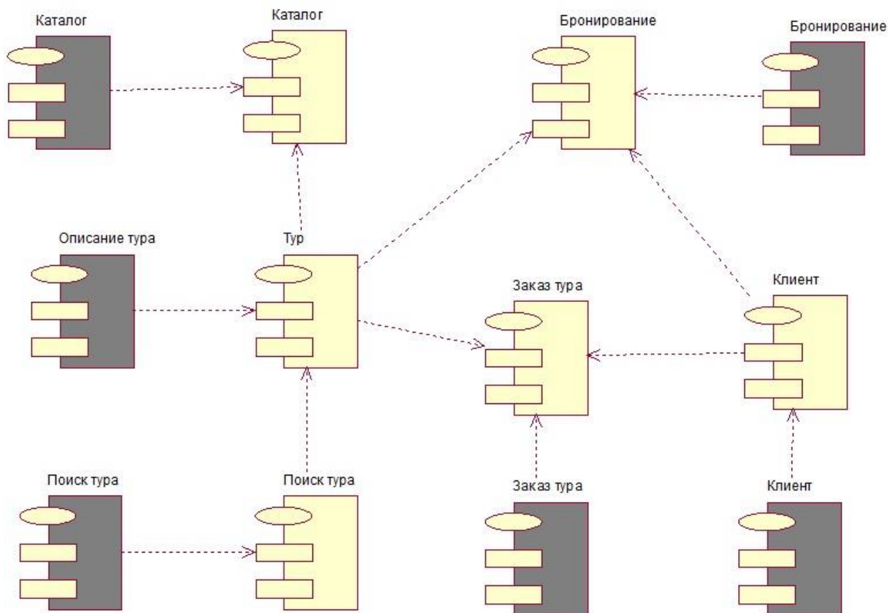
Рис. 9.3. Диаграмма компонентов предметной области «Туристическое агентство»
