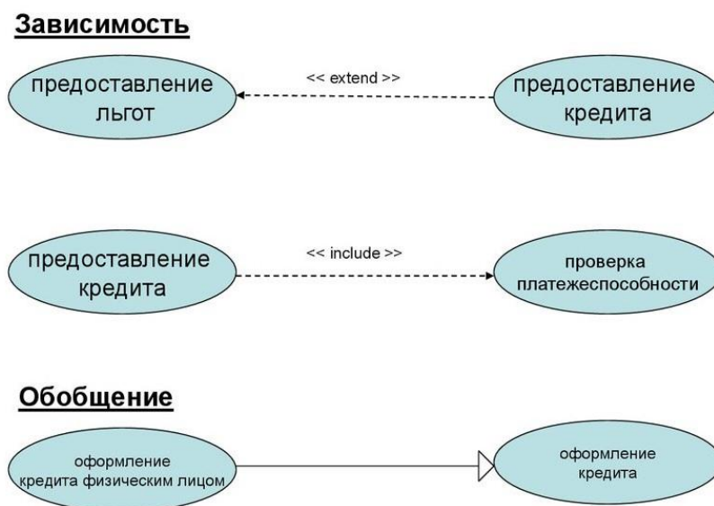
Рис. 5.1. Обозначение связей между прецедентами
