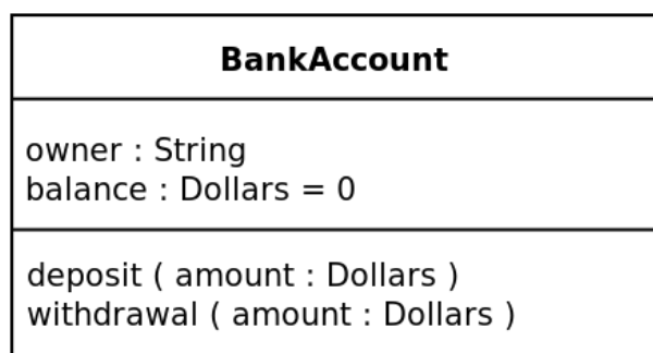
Рис. 6.1. Класс с двумя методами полями
